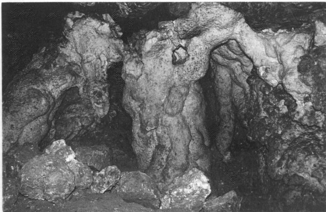
"Fatörzsek" - gipszoszlopok a Sátorkőpusztai-barlang Benedek-termében
