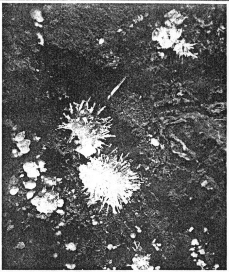
ARAGONITTŰK Beremendi kristálybarlang
