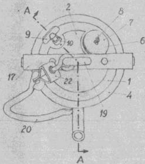
FELÜLNÉZET
