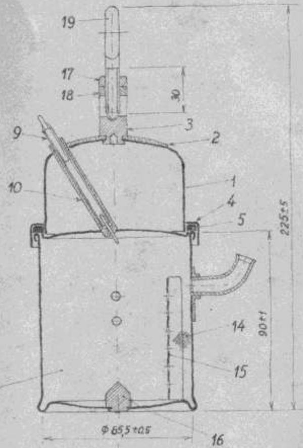
"A" - METSZET
