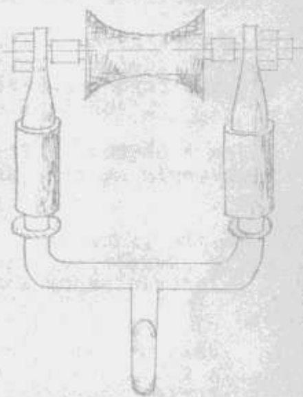
OLDALGÖRGŐS AUTÓMÁTUS /VÁCSÓ KERET/
